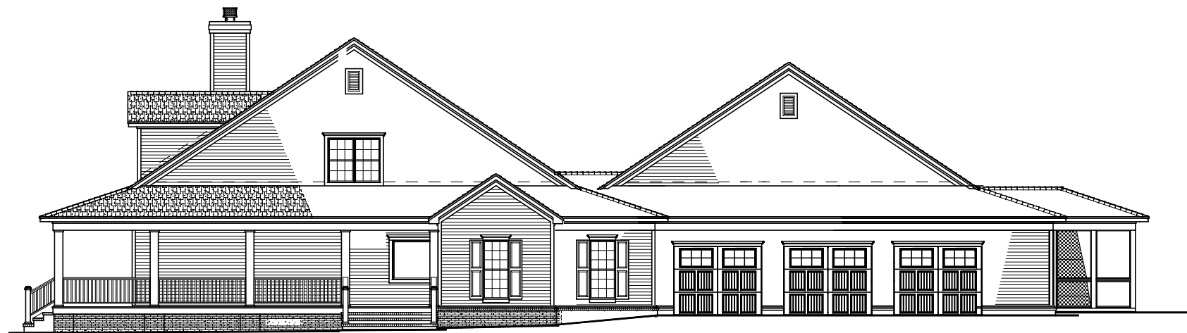
RIGHT ELEVATION
